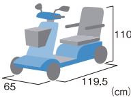
重量:101kg 連続走行距離:28km 耐 100kg
