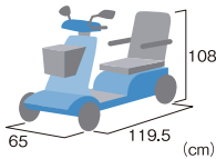
重量:97kg 連続走行距離:30km 耐 100kg
