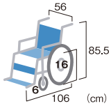
重量:16.9kg(バッテリー含まず) 連続走行時間:約130分 連続走行距離:7km 耐 75kg
