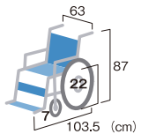
重量:32.3kg 充電時間:約2～3時間 連続走行距離:16km 耐 100kg
