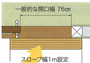
車いすで斜めに入りやすいよう、 スロープ幅を広く設置
